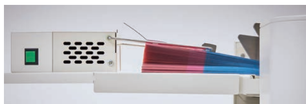
エアースタバキユニットで用紙がさばかれている状態
