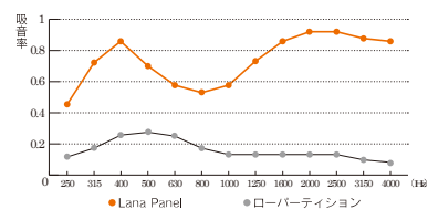
■残響室法吸音率測定より
