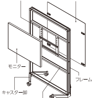
ラダー ※モニタータイプは3本、標準タイプは2本になります。
