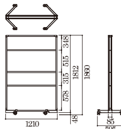
1812モニタータイプ
